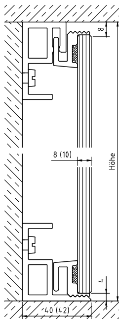
Standardbefestigungssystem
