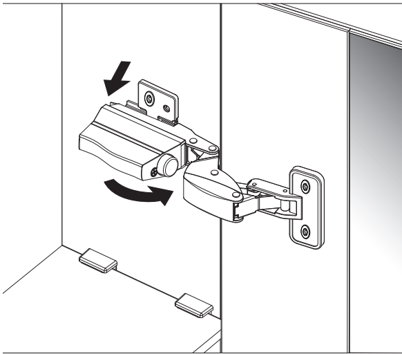
Scharnier mit Dämpfung
